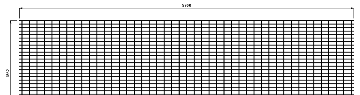
STEROP2 - 62x32 - 25x2 - Ø4,5
