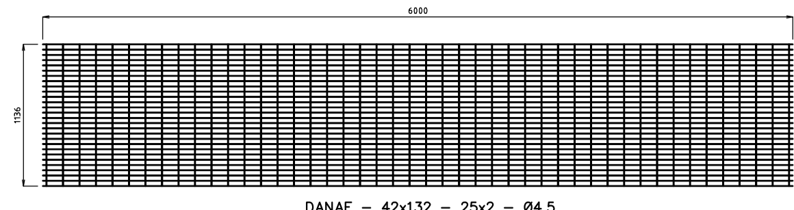
DANAE - 42x32 - 25x2 - Ø4,5
